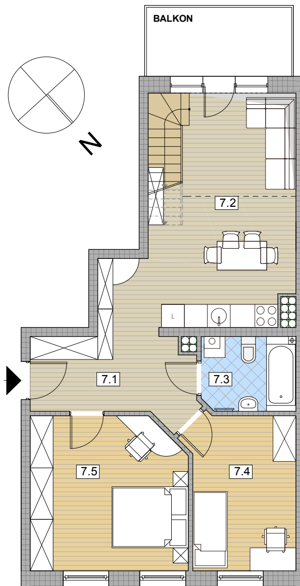
C11 - POZIOM DOLNY - ARANŻACJA II 66,10 m 2
